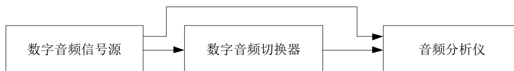
图3 输入接口最大输入电压测量框图
