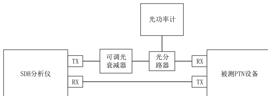
图12 接收机灵敏度测量框图
