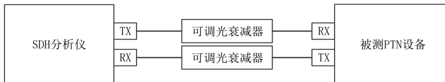
图18 误码测量框图
