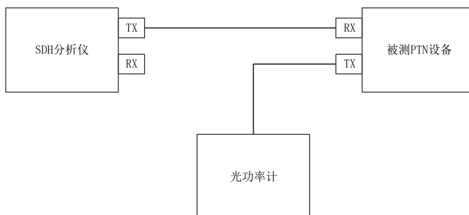
图9 平均发送光功率测量框图
