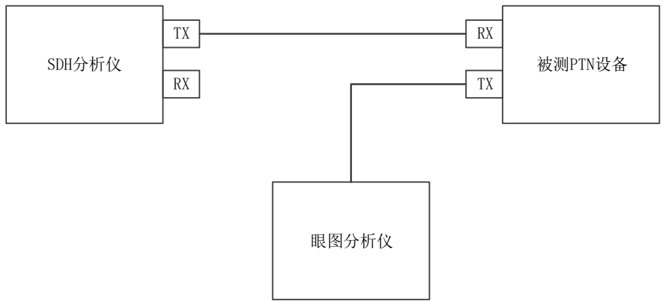
图10 消光比、发送信号波形测量框图
