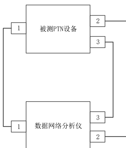
图15 MAC 地址黑名单、风暴抑制、镜像功能测量框图
