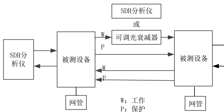
图19 网络管理测量框图
