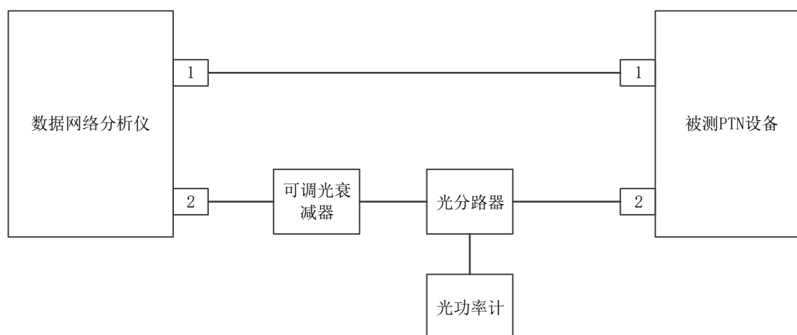
图6 接收灵敏度测量框图
