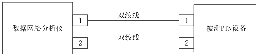
图7 接口传输距离、半双工-全双工自动协商测量框图
