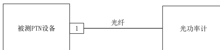
图3 平均发送光功率测量框图
