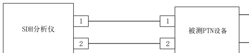
图8 输出信号时钟、输出口抖动测量框图
