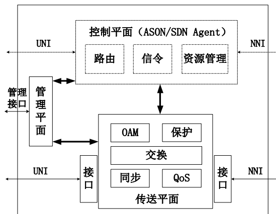
图1 接入型 PTN 设备系统结构框图
